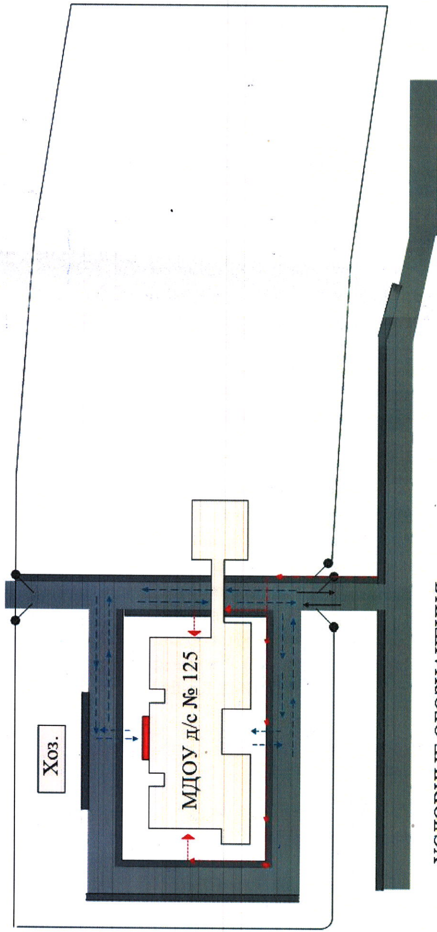
1.3. План-схема путей движения транспортных средств к местам разгрузки/погрузки и рекомендуемых безопасных путей передвижения воспитанников, их родителей (или законных представителей) по территории МДОУ д/с № 125
